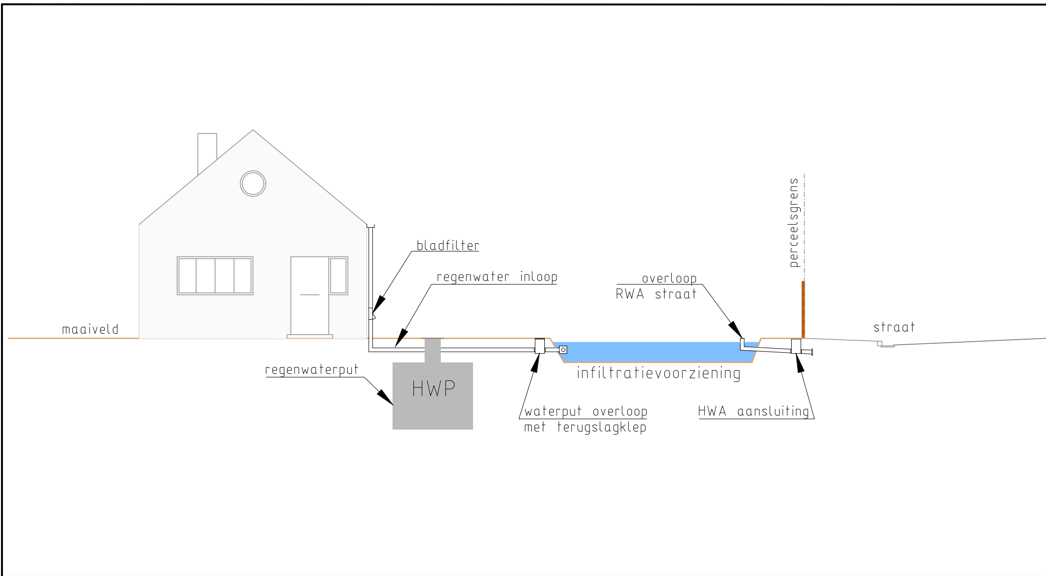
Typetekening RWA met waterput en overloop
